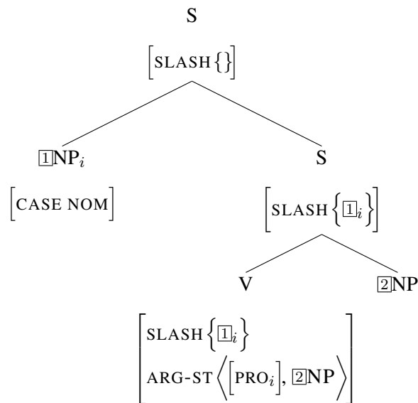
Figure 3: SVO
